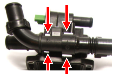
Montaje Termostato y Tubo
