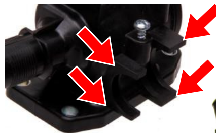
Termostato 1336-V3
